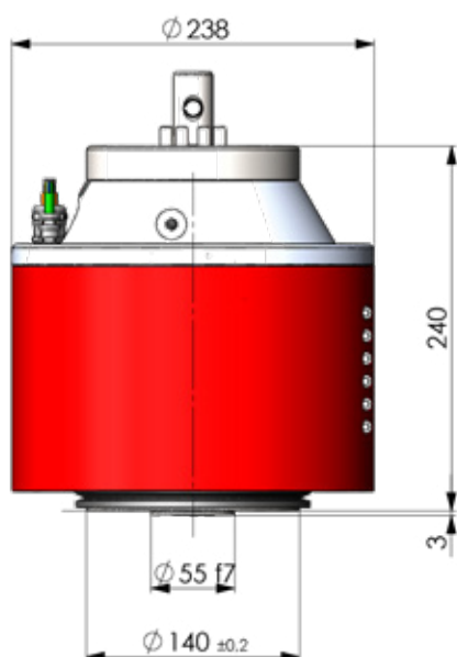
BV140 - Dimensions
